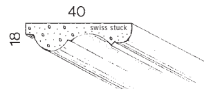
▲ P073 12×40mm
