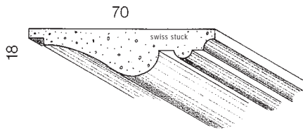
▲ P050 18×70mm
