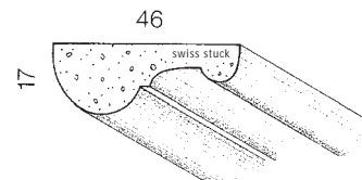
▲ P076 17×46mm ▲ P074 25×65mm ▲ P075 22×55mm ▲ P077 14×35mm
